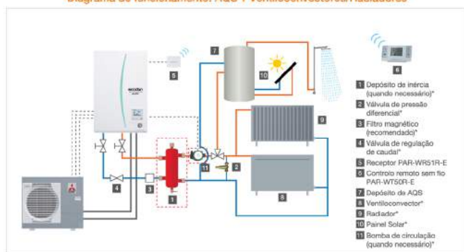
Diagrama de funcionamento: AQS + Ventiloconvectores/Radiadores
