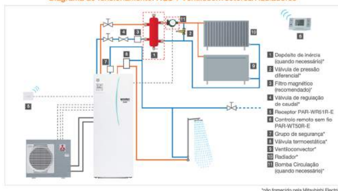
Diagrama de funcionamento: AQS + Ventiloconvectores/Radiadores
