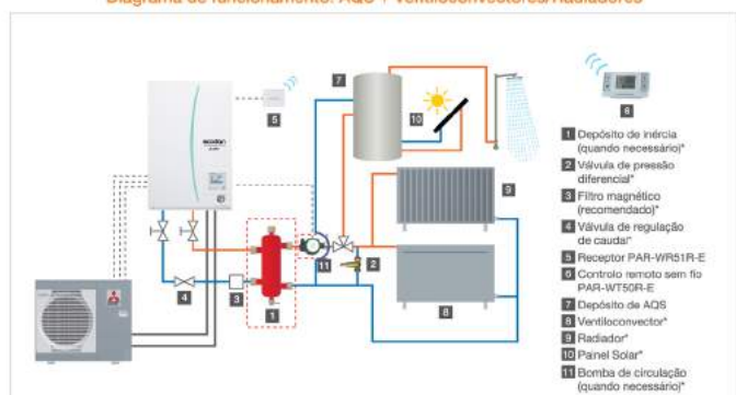
Diagrama de funcionamento: AQS + Ventiloconvectores/Radiadores
