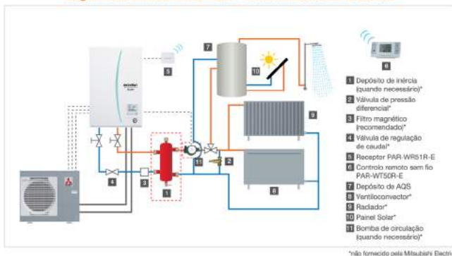
Diagrama de funcionamento: AQS + Ventiloconectores/Radiadores
